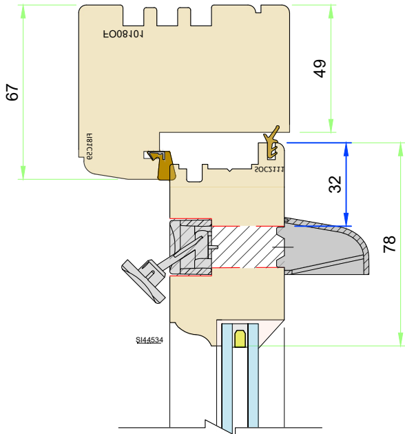
Sash vent Scale 1:2
