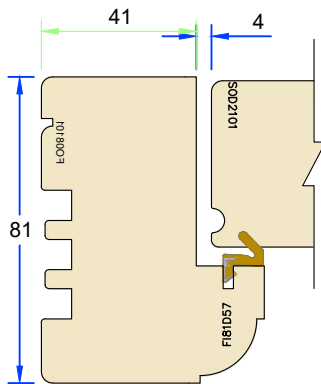
81mm frame – Ovolo profile
