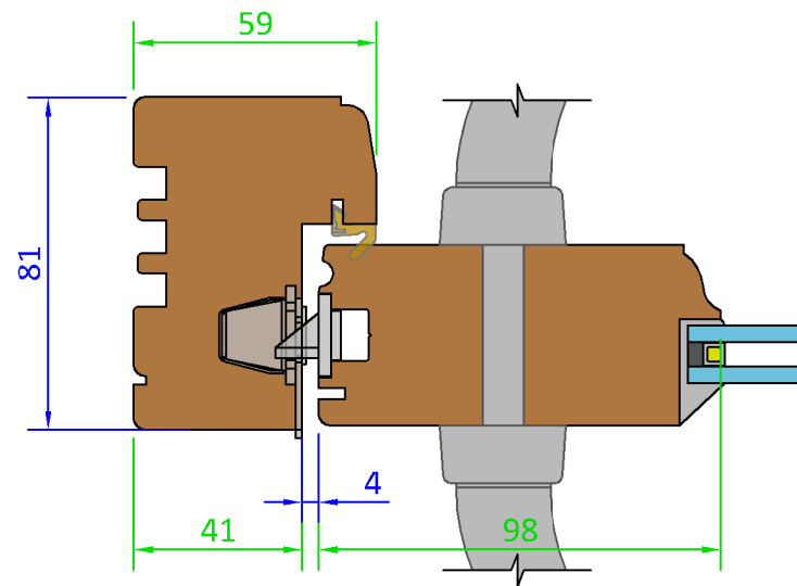
Section A-A - Jambs (Scale 1:2)
