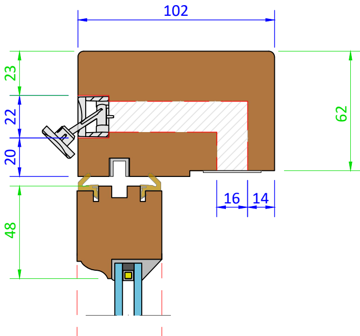
Vent Option - (Scale 1:2)
