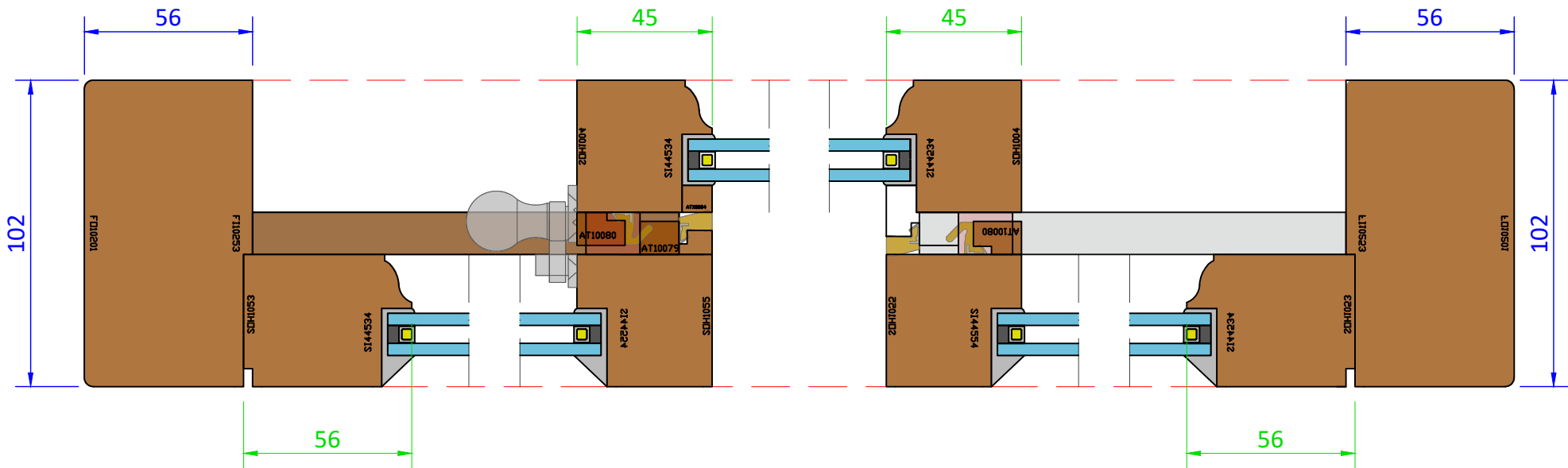
Section D-D - (Scale 1:2)
