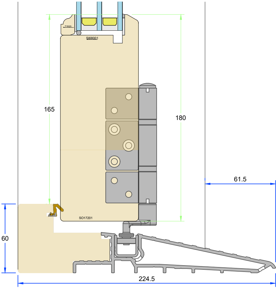
Section C-C - Jamb detail
