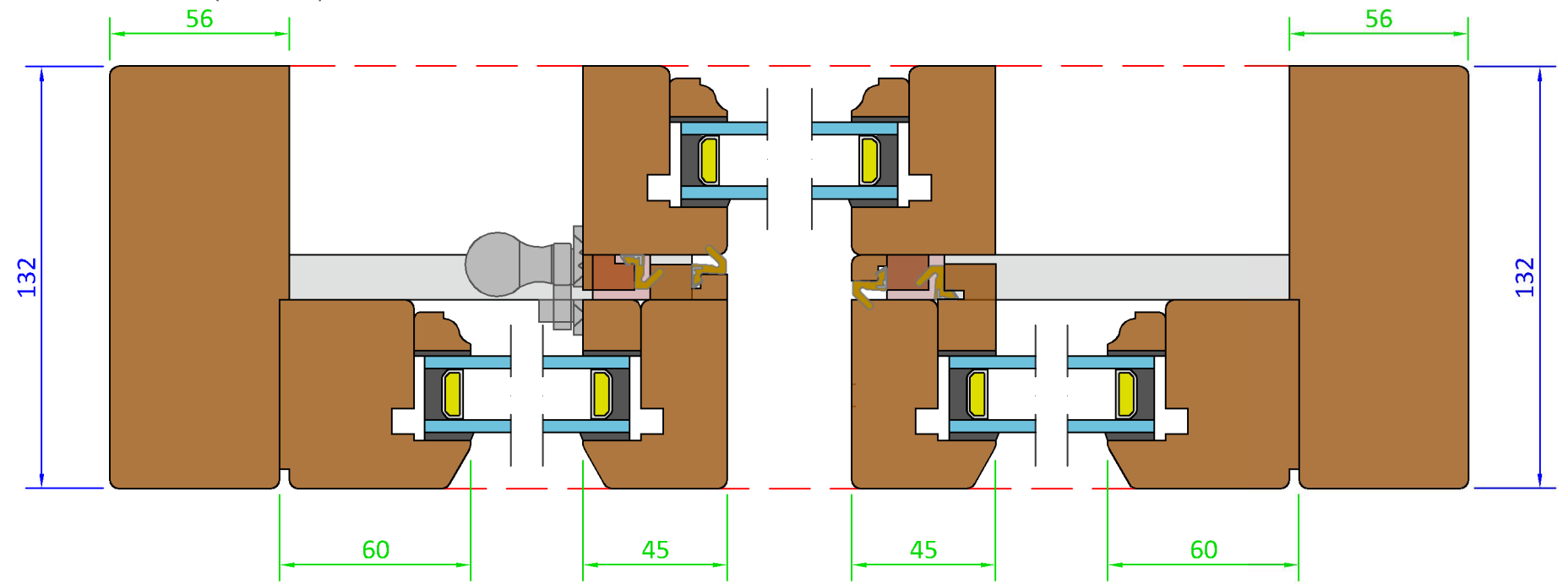
Section D-D - (Scale 1:2)
