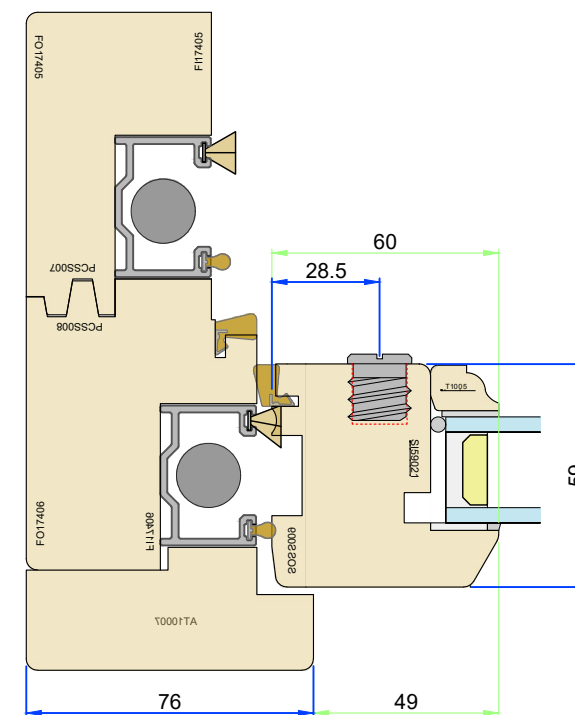
Section B-B - Upper Jamb
