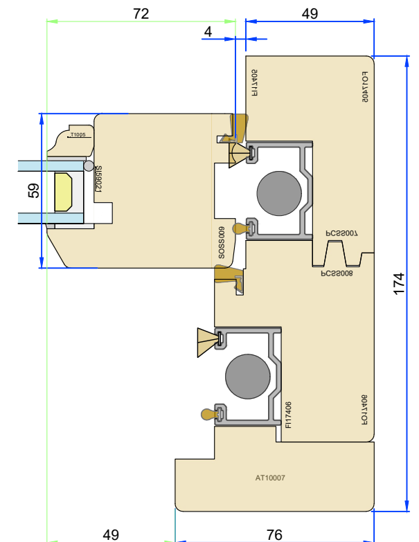
Section C-C - Lower Jamb
